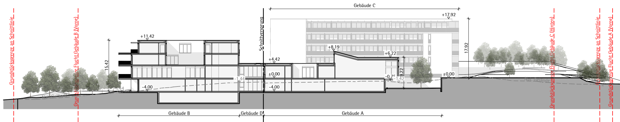
Schnitt B-B
