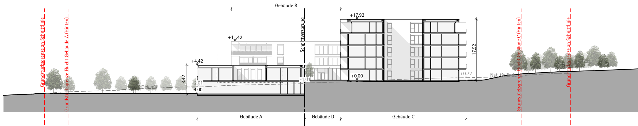
Schnitt A-A
